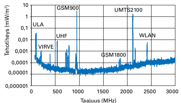
Kuva 6. Esimerkkspektri kaupungissa sijaitsevan kerrostalon ylimmässä kerroksessa suoritettua mittauksesta. Kerrostalon katolle on asennettu matkapuhelintukiaseman antenneja. Matkapuhelinjärjestelmien aiheuttamien taajuuskomponenttien lisäksi spektrissä näkyvät radio- ja TV-lähetykset (ULA, VHF), TETRA-tekniikalla toteutetun viranomaisverkon (VIRVE) ja langattoman verkon (WLAN) aiheuttamat komponentit.
