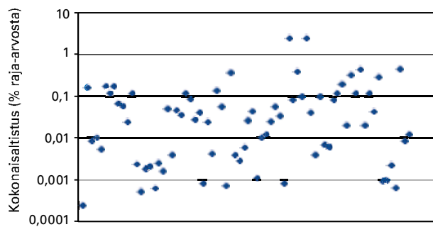
Kuva 4. Matkapuhelinjärjestelmien aiheuttama kokonaisaltistus mittauskohdeissa
