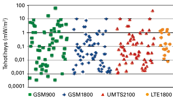
Kuva 5. Eri matkapuhelinjärjestelmien aiheuttamat tehotiheydet mittauskohdeissa
